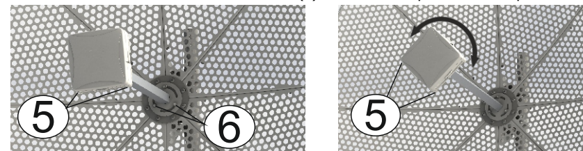
Рисунок 4 – Начальное положение облучателя с поляризацией X-pol (слева) и V+H (справа, при этом более короткий кабель облучателя соответствует вертикальной поляризации, а более длинный - горизонтальной)
